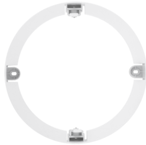
Soporte de montaje de superficie FR12 para LED downlights PR1240 y PR12CCT
